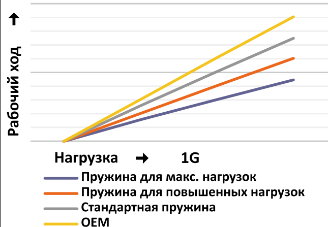
Рабочие характеристики пружин OBK
